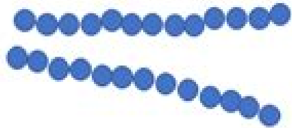
Linear Polymers
